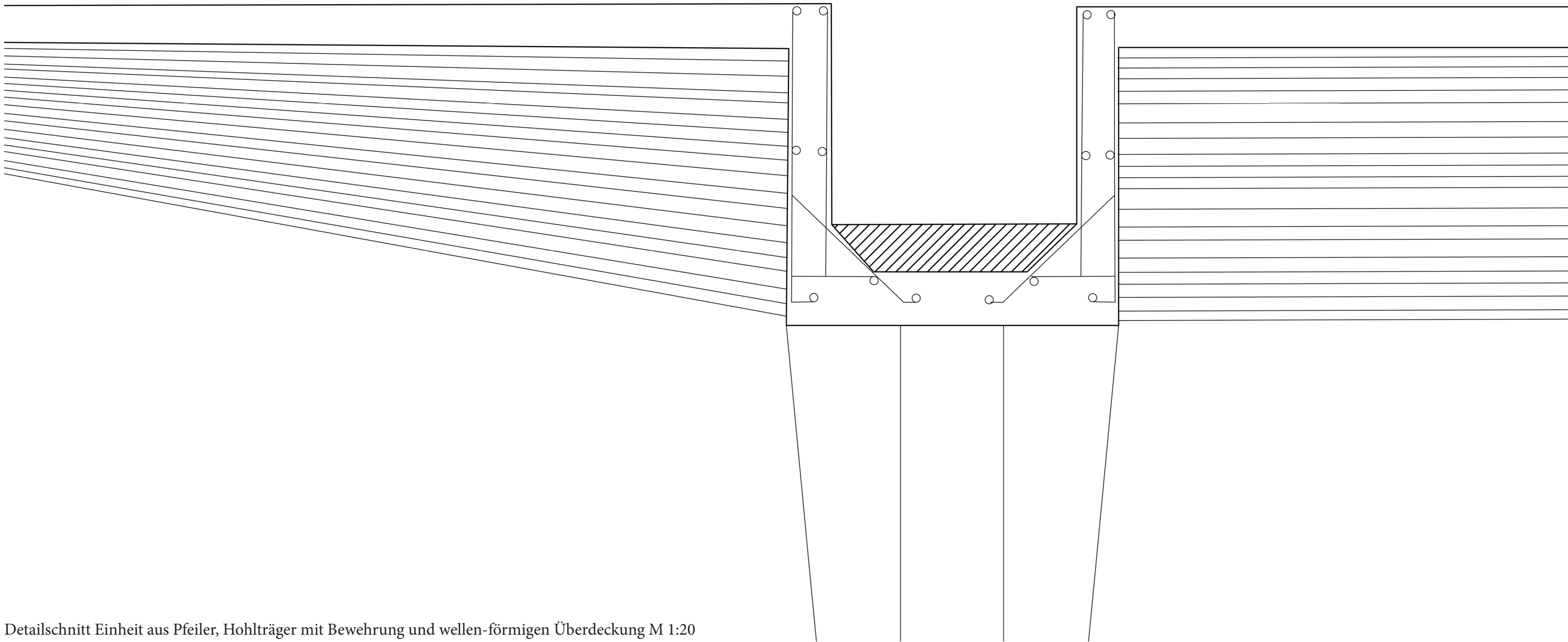
Detailschnitt Einheit aus Pfeiler, Hohlträger mit Bewehrung und wellen-förmigen Überdeckung M 1:20
